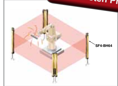
Schutzraum um Schweißroboter
